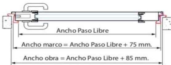
Vista de Planta
