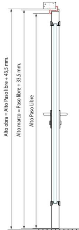
Vista de Perfil
