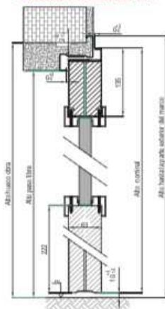
Sección Vertical A-A
