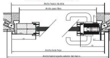
Sección Horizontal B-B
